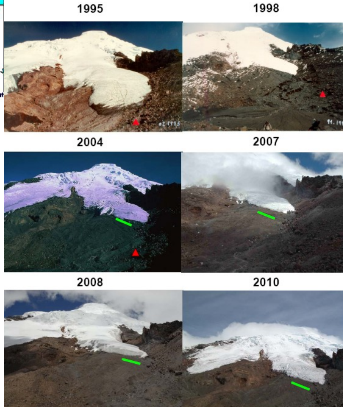
Glaciar 15 Volcán Antisana Ecuador
